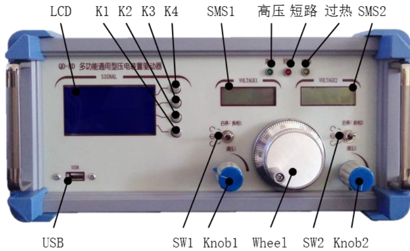
前面板
