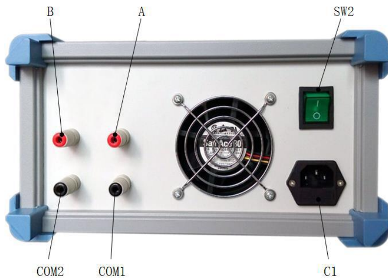
后面板
